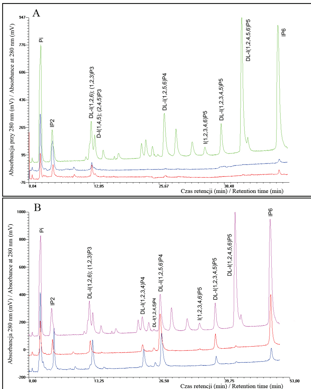
Rys. 4. Profile chromatograficzne fosforanów mio -inozytoli w enzymatycznie modyfikowanym cieście A. 60. minuta fermentacji: chromatogram referencyjny: termiczny hydrolizat kwasu fitynowego (—); pieczywo z dodatkiem 3-fitazy A [1500 FTU/kg mąki] (—); pieczywo z dodatkiem 3-fitazy A [1500 FTU/kg mąki] oraz kwaśnej fosfatazy [30 AcPU/ g mąki] (—). Analiza metodą HPLC B. 150 min fermentacji: chromatogram referencyjny: termiczny hydrolizat kwasu fityno-
